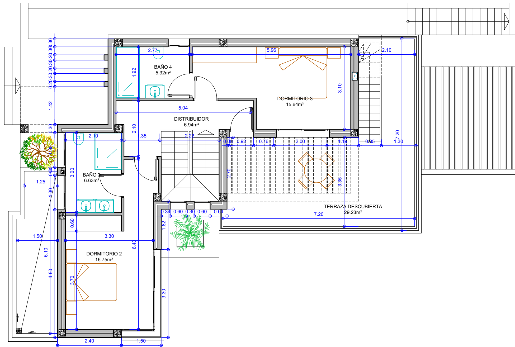
PLANTA PRIMERA
