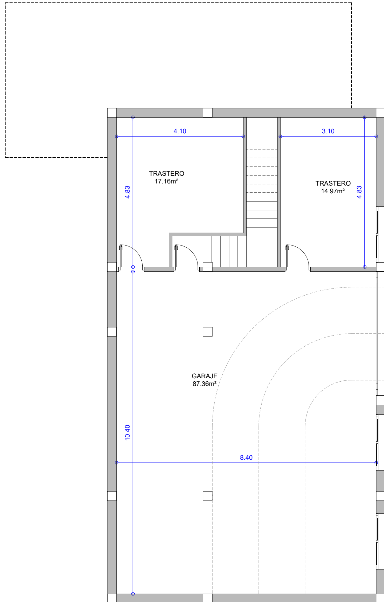
PLANTA SEMISÓTANO Sup. Construida = 143.82m 2
